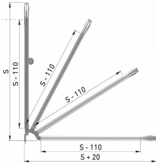
Codo
