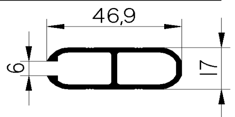
Perfil capota
